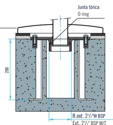
Detalle anclaje Anchor detail
