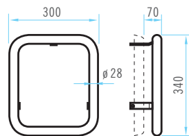
Rectangular em inox AISI-316 pintado (Cód. 09447) S.S. AISI-316 square painted (Cod. 09447)
