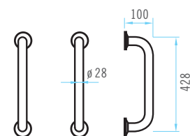
Dupla em inox AISI-316 polido (Cód. 05557) S.S. AISI-316 polished for twin faceplate (Cod. 05557)
