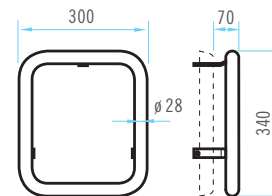
Rectangular em inox AISI-316 polido (Cód. 00246) S.S. AISI-316 Square polished (Cod. 00246)
