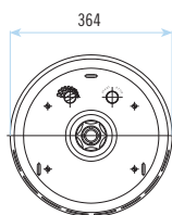
Plástico branco para caixa de alojamento em inox (Cód. 11500) White ABS for S.S. wall housing. (Cod. 11500)
