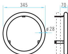
Redonda em inox AISI-316 pintado (Cód. 07536) S.S. AISI-316 round painted (Cod. 07536)
