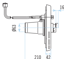
Plástico branco para caixa de alojamento em inox (Cód. 11500) White ABS for S.S. wall housing. (Cod. 11500)
